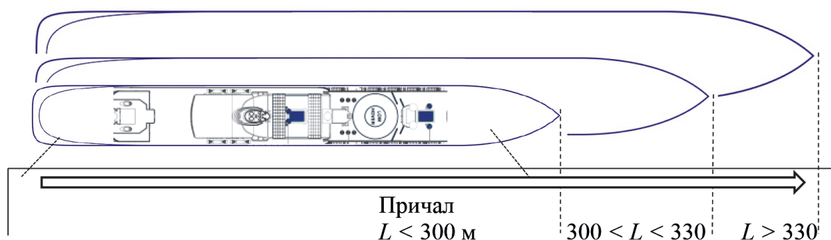
Рис. 1. Параметры для увеличения размеров круизных и паромных судов и причалов: L — длина круизного / паромного судна
